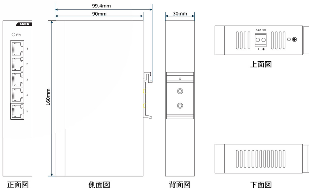
寸法図
