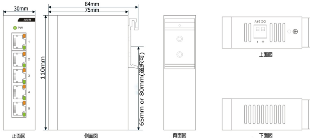
寸法図
