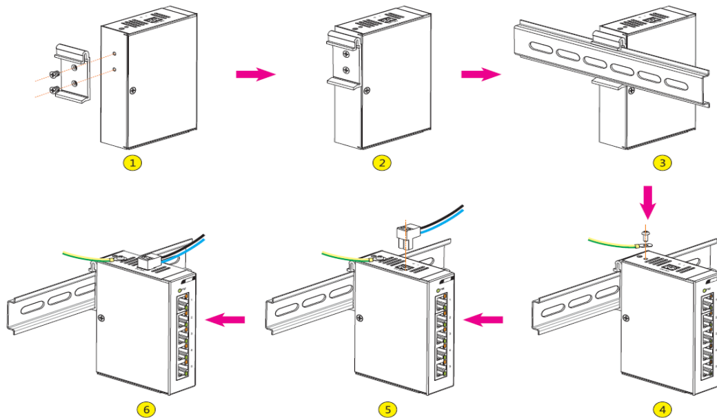
取付手順図
